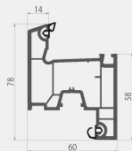
012 Штульп
