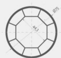
014 З'єднувач-підсилювач
