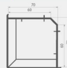
075 Н-з'єднувач рами
