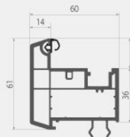
012 Штульп
