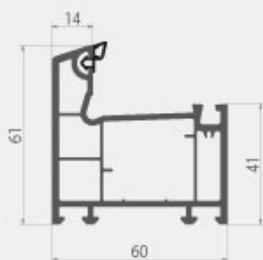
017 Рама 3-камерна
