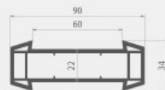
014 З'єднувач-підсилювач
